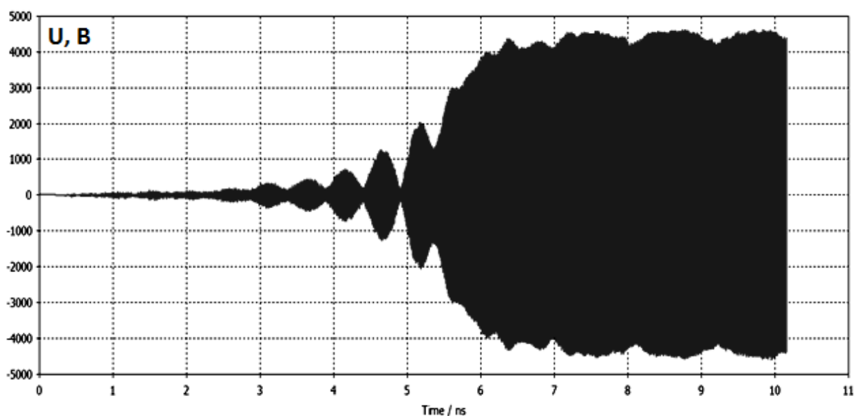
Рис.5 - Процесс возбуждения колебаний для колебательной системы с 6 неоднородностями с выводом энергии в резонаторе А
