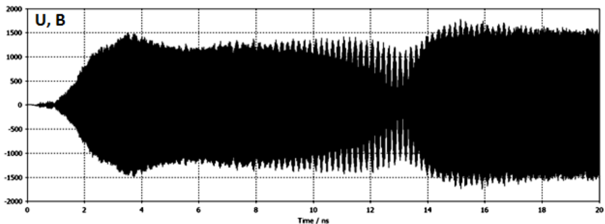
Рис. 6 - Процесс возбуждения колебаний для колебательной системы с 6 неоднородностями с выводом энергии в резонаторе В
